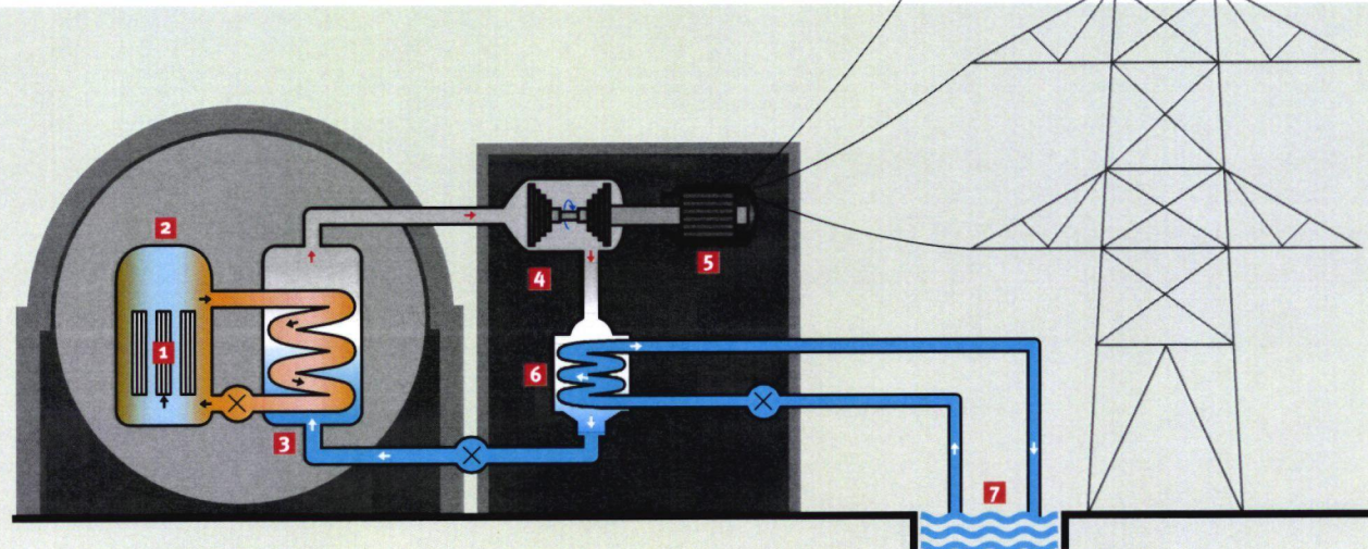
Figuur 2.2.1 Principeschema van de installatie
