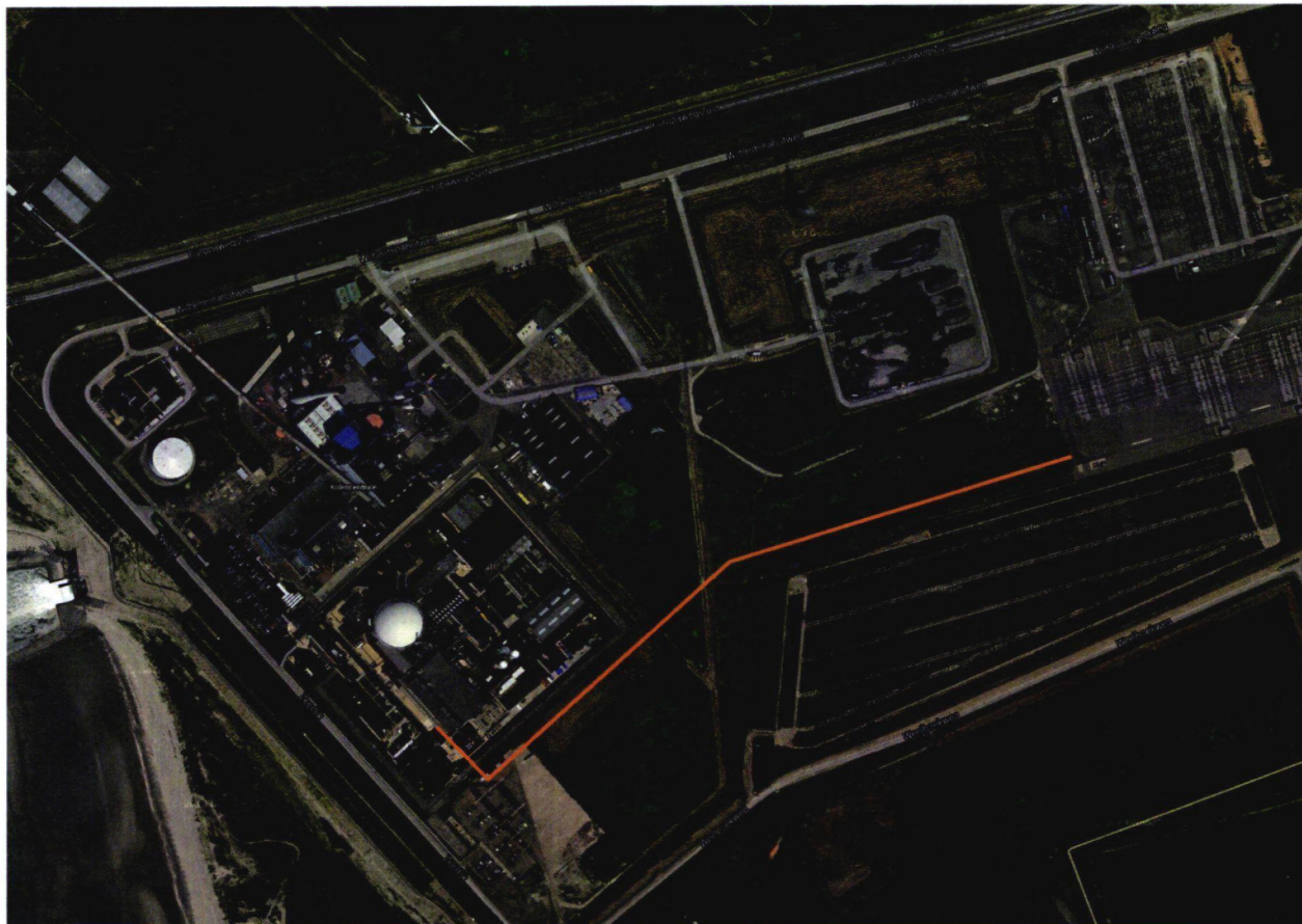
Figuur 2.3.8.1 Globaal overzicht kabeltracé (aangegeven in oranje)
