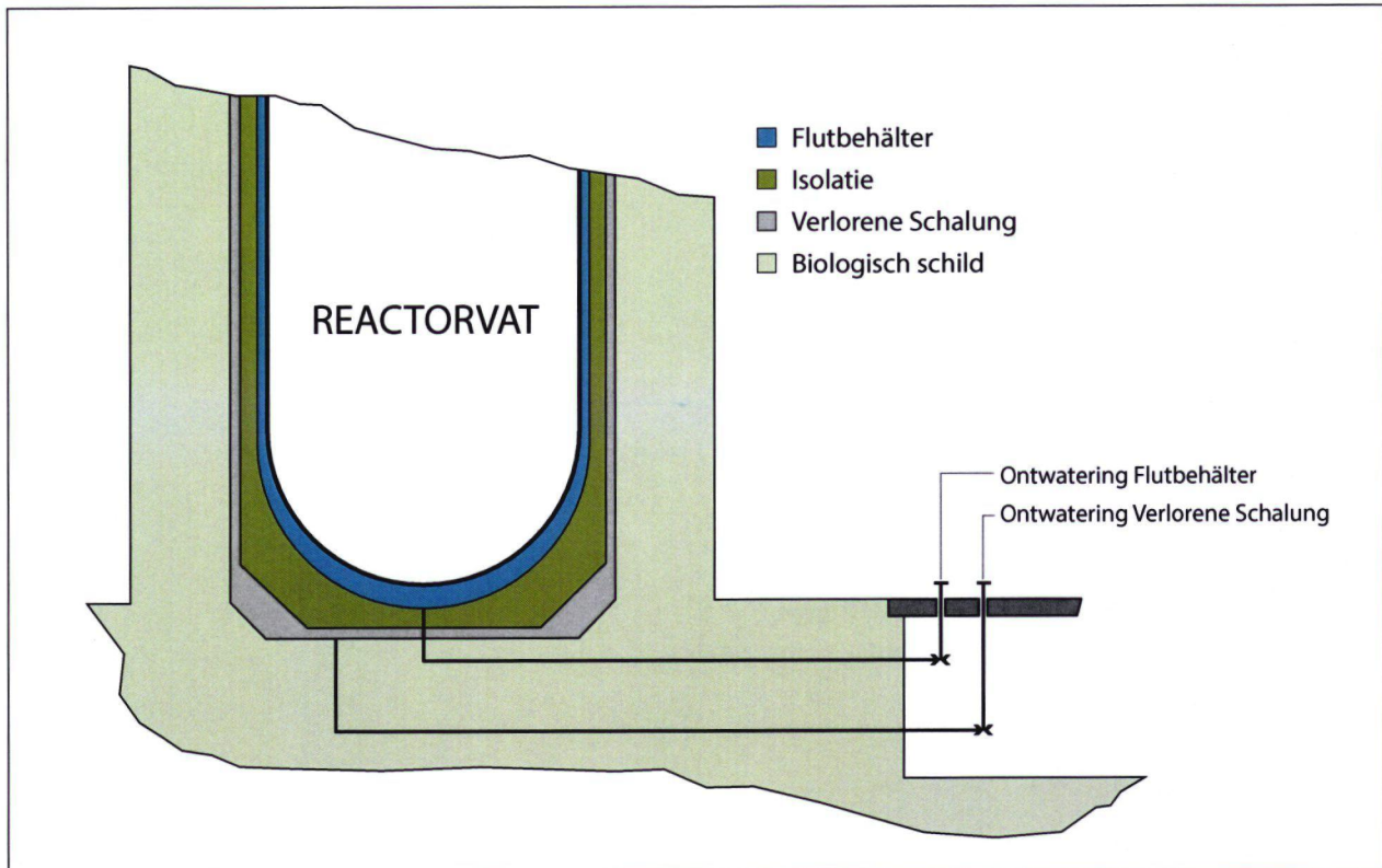
Figuur 2.3.9.1 Doorsnede van reactorvat en Flutbehälter
