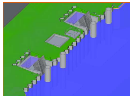
Afbeelding 2 - Bovenaanzicht van inname punten incl. waterlijn (uit 3D-model)
