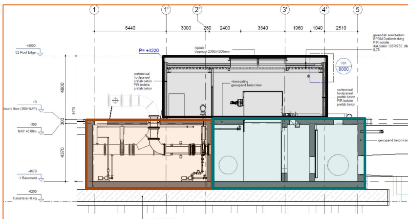
Afbeelding 7 - Doorsnede pompgebouw (oranje = droge kelder; groen = natte kelder; grijs = bovenbouw)
