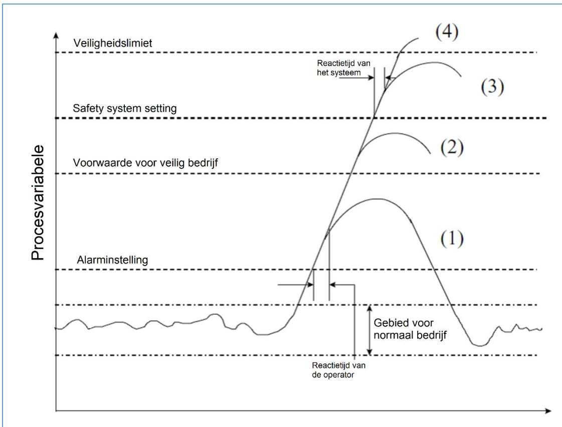
Figuur 18-1: Schema van veiligheidslimieten en instellingen van de veiligheidssystemen (Safety system settings)
