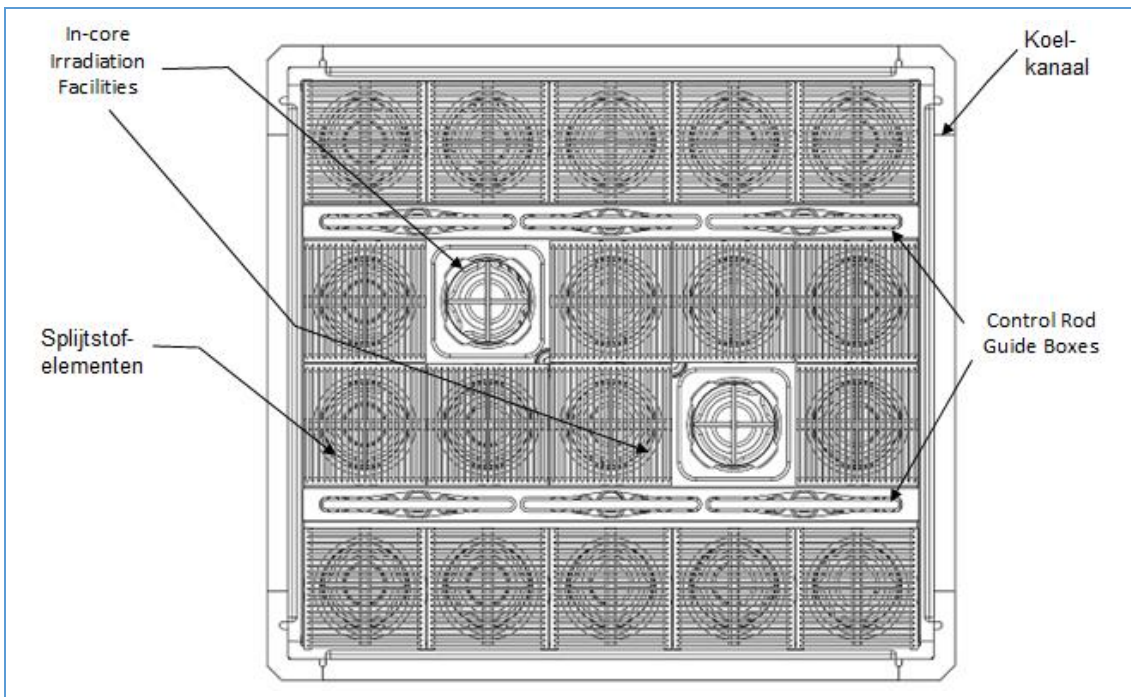
Figuur 5-3: Bovenaanzicht van de PALLAS-reactorkern, kernconfiguratie met 18 splijstofelementen
