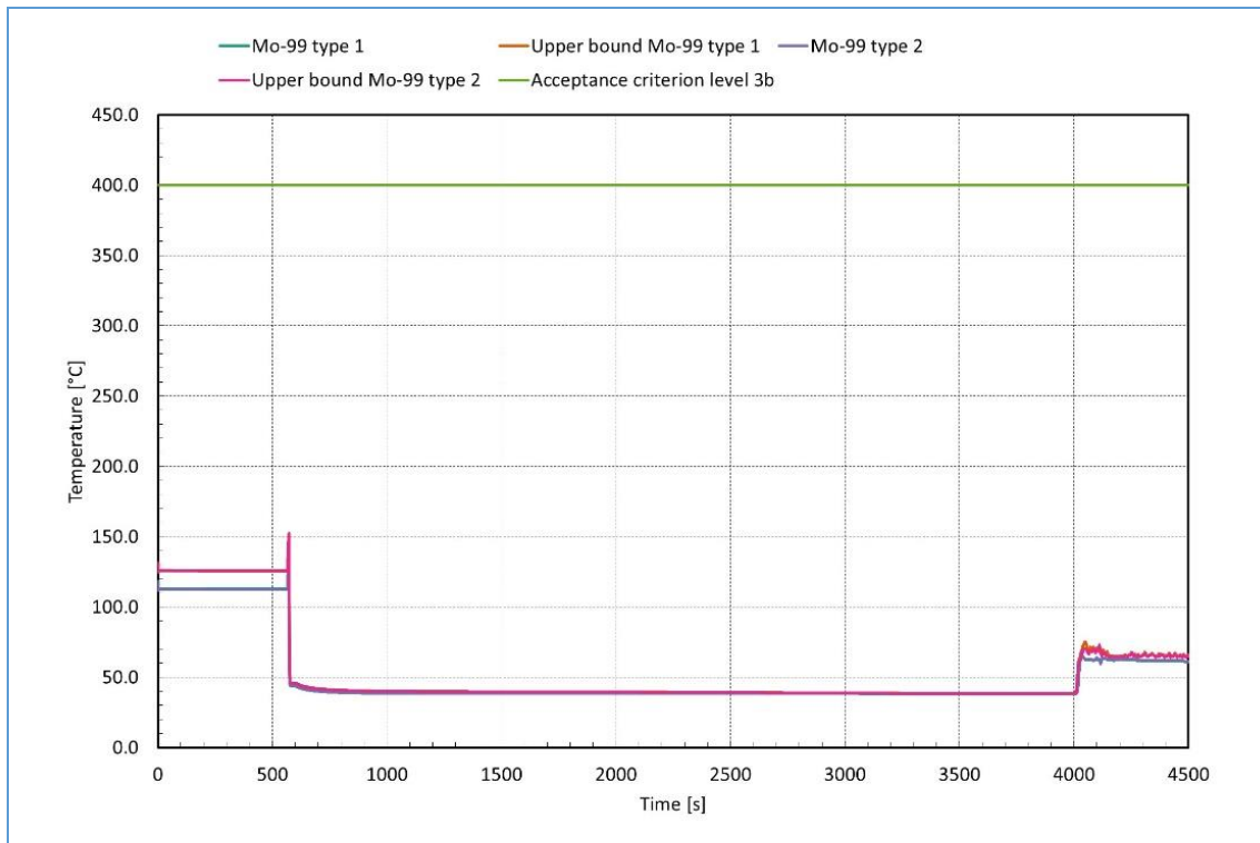
Figuur 16-43: Temperatuur van de bekleding van de Mo-99 targets - PIE-079
