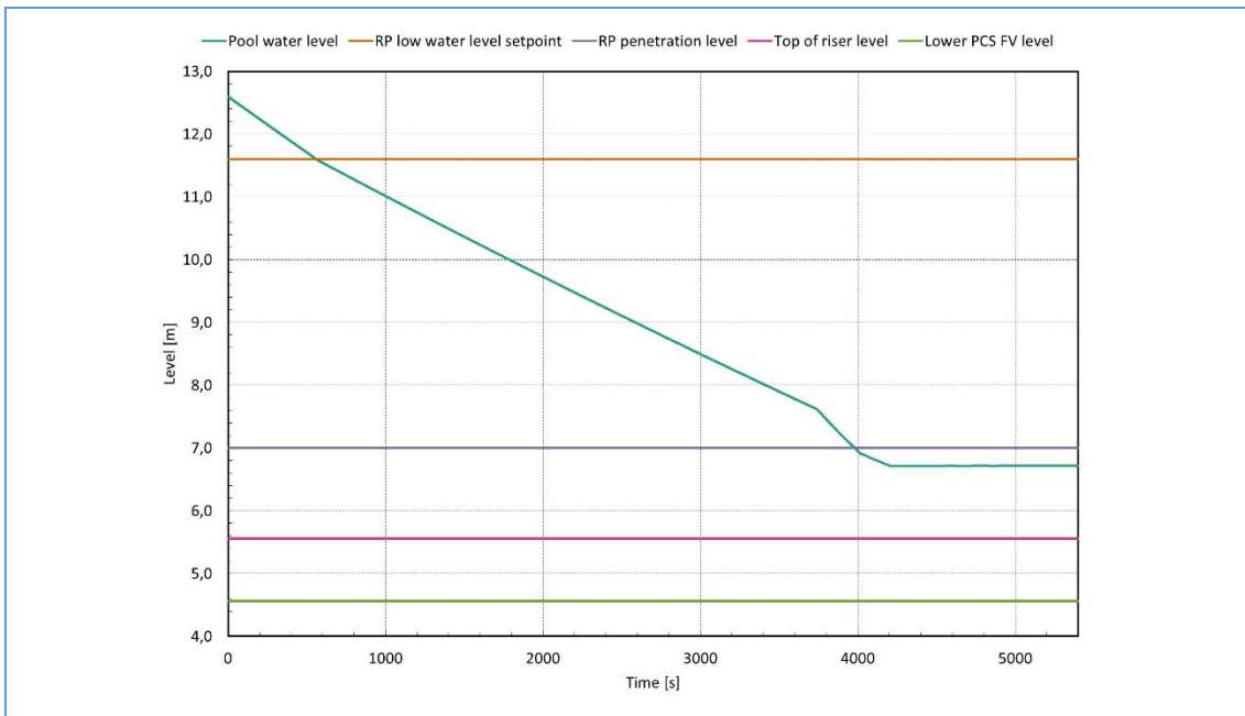
Figuur 16-7: Waterniveau in de Reactor Pool, PIE-009
