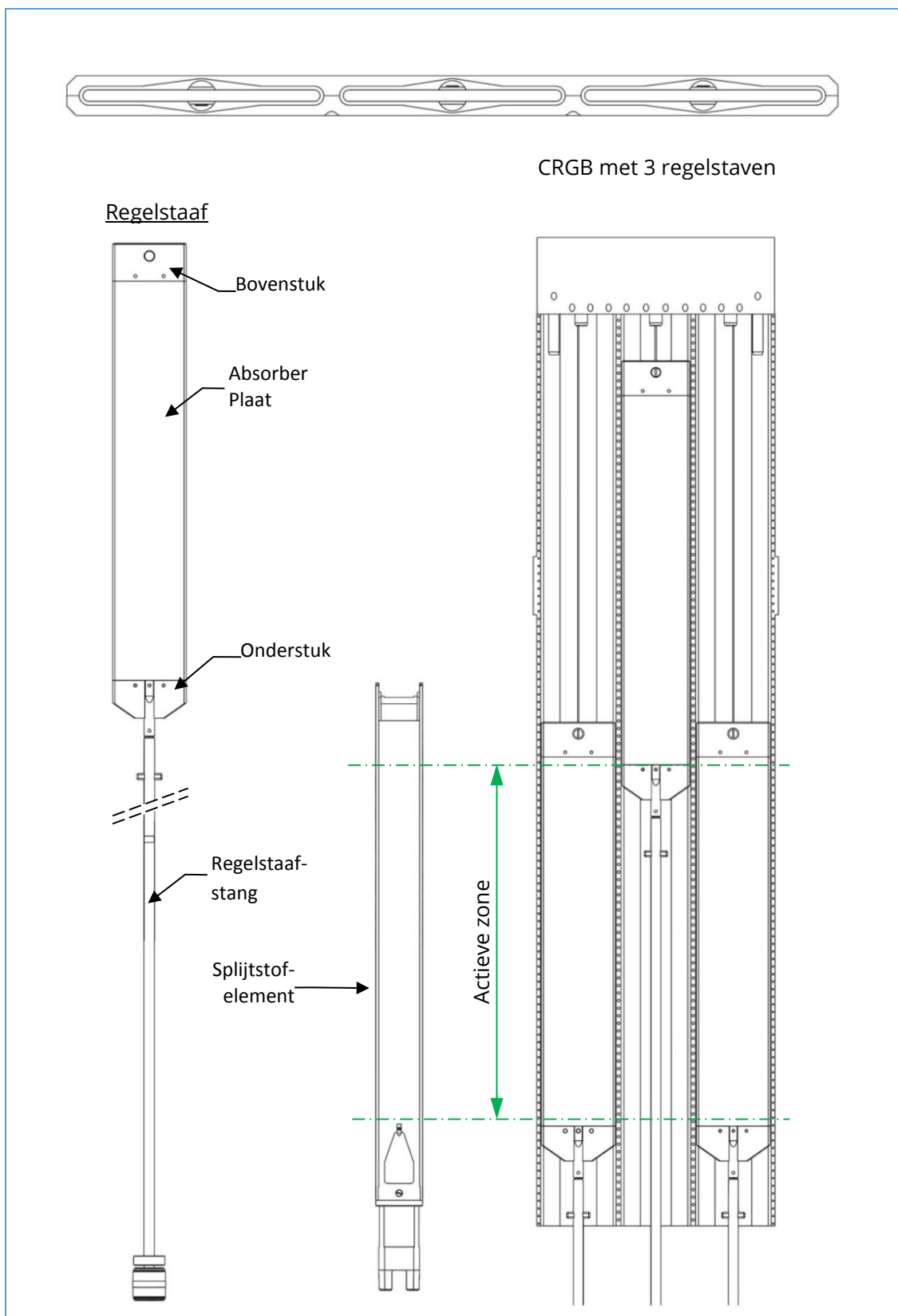
Figuur 5-12: CRGB en regelstaven (figuur is ter illustratie waarbij details kunnen afwijken)
