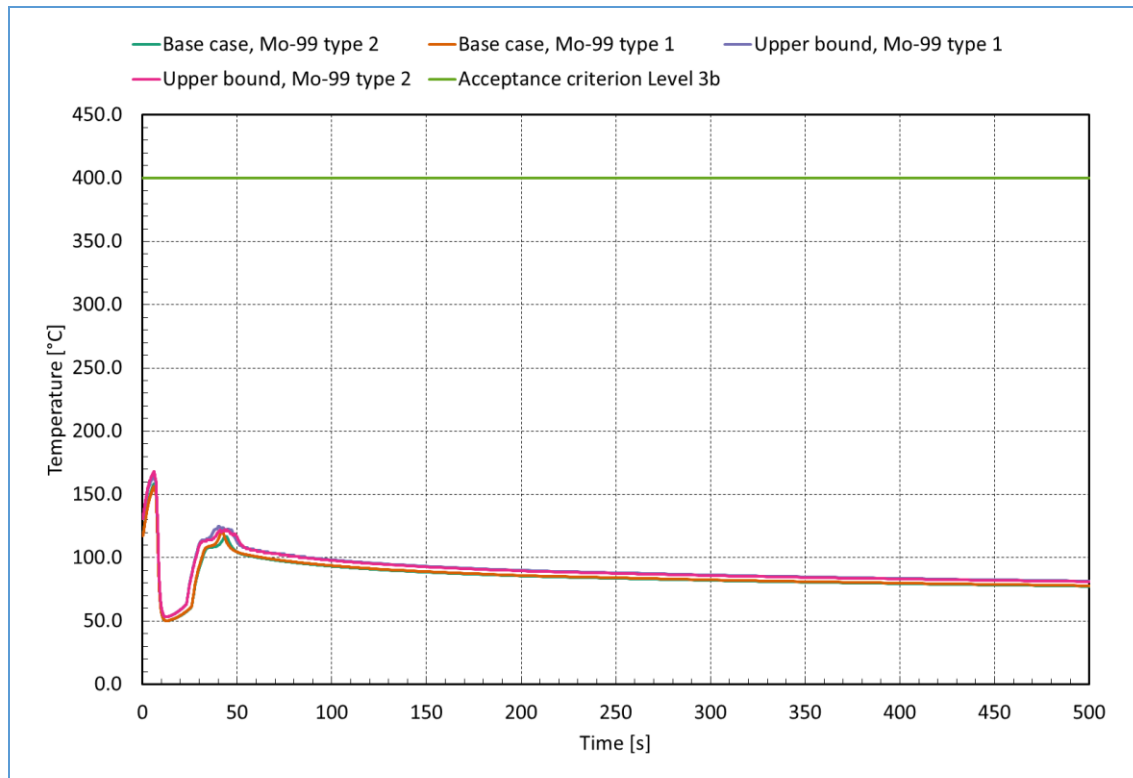
Figuur 16-38: Temperatuur van de bekleding van de Mo-99 targets – PIE-071
