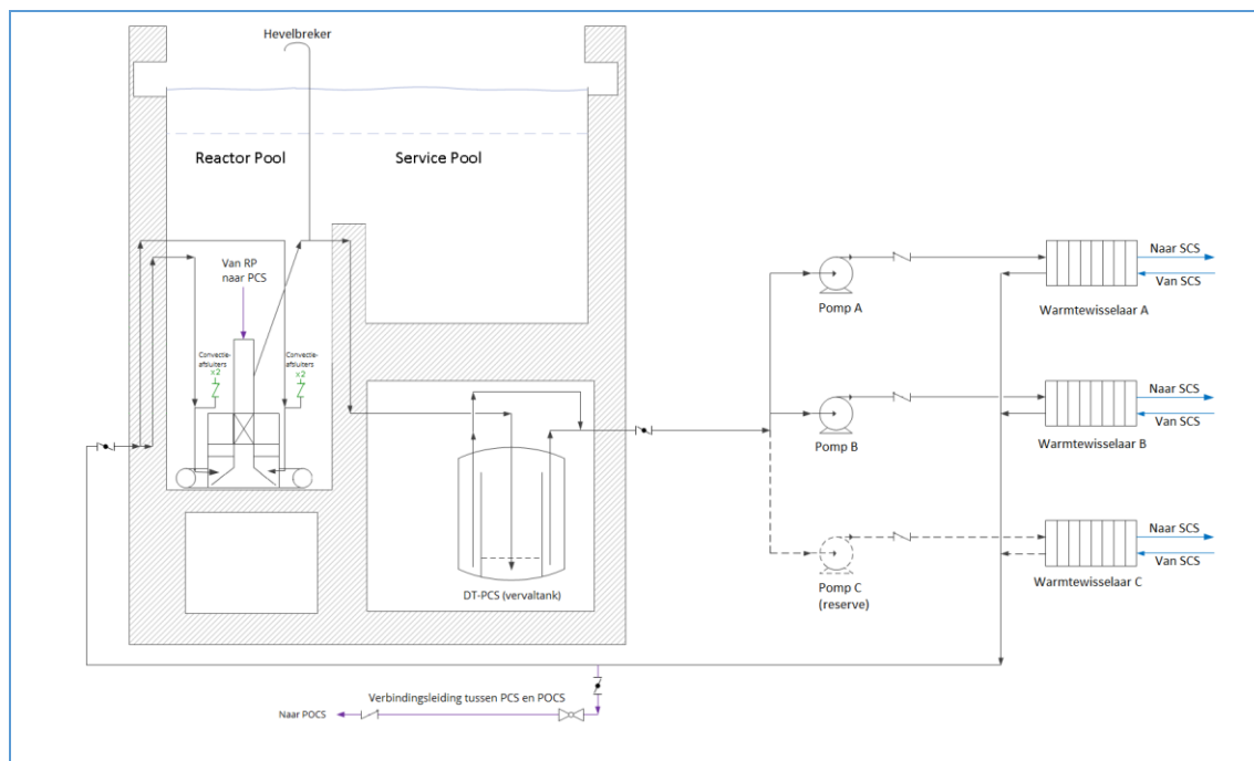
Figuur 6-2: Vereenvoudigd PCS-processtroomdiagram (Reactor in vermogenstoestand)
