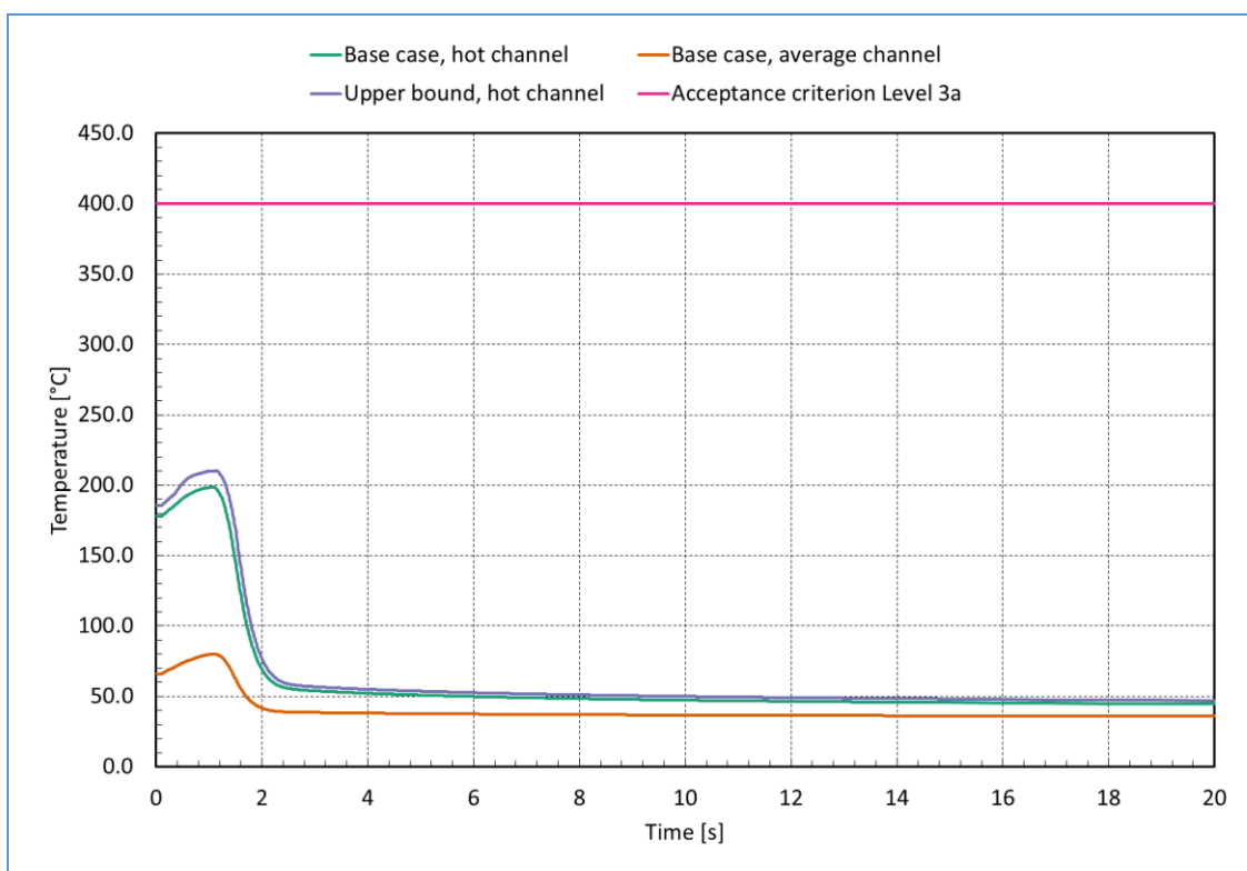
Figuur 16-13: Temperatuur van de bekleding van de splijststofelementen - PIE-016
