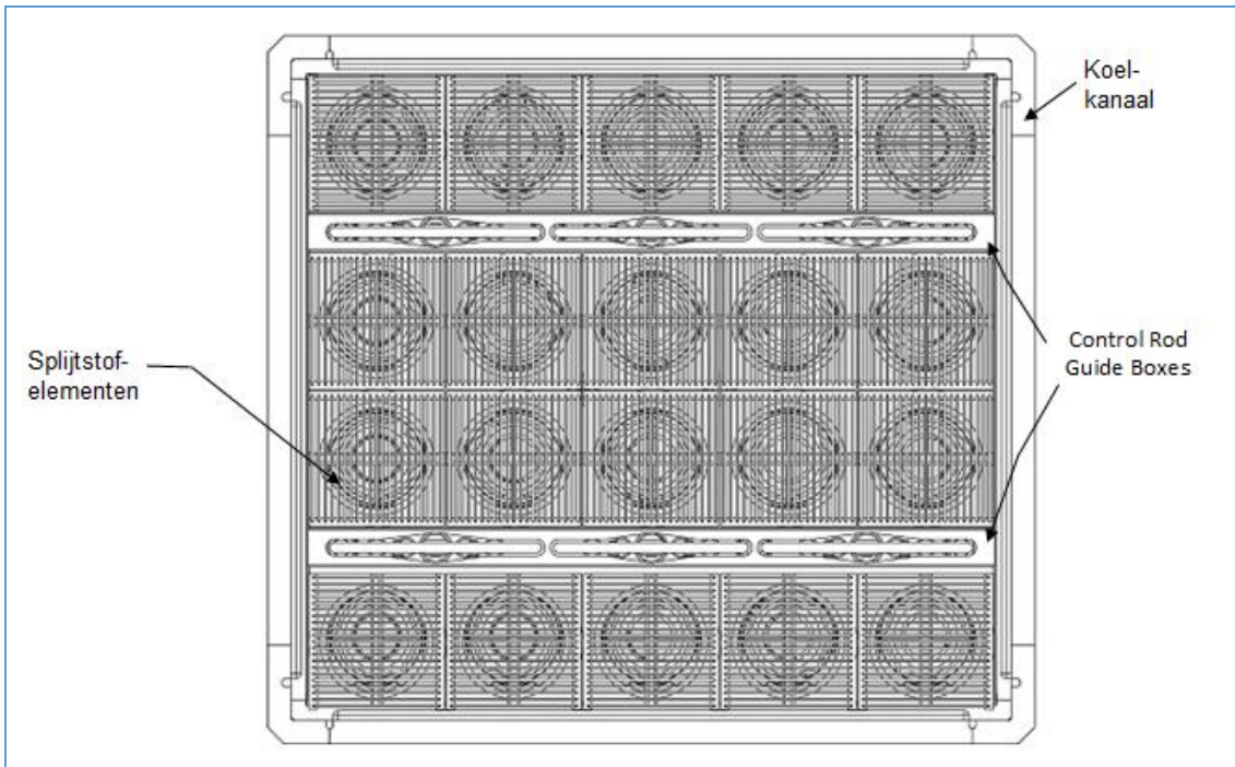
Figuur 5-2: Bovenaanzicht van de PALLAS-reactorkern, kernconfiguratie met 20 splijstofelementen
