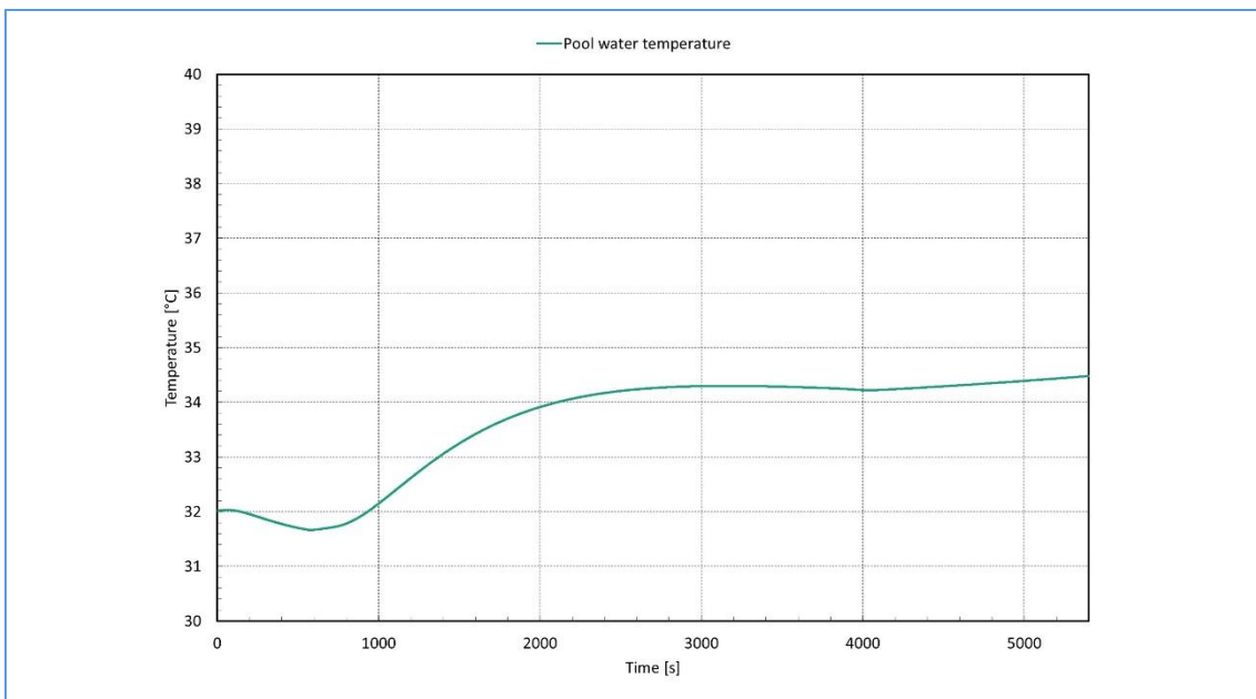
Figuur 16-8: Temperatuur van de Reactor Pool, PIE-009
