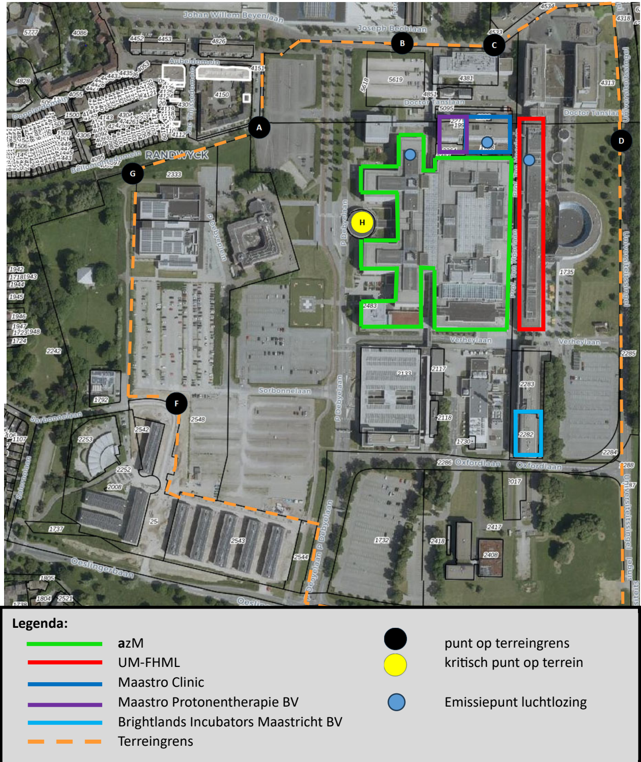
Figuur F-1: Terreingrens Complex Randwyck ten behoeve van stralingsbescherming.
