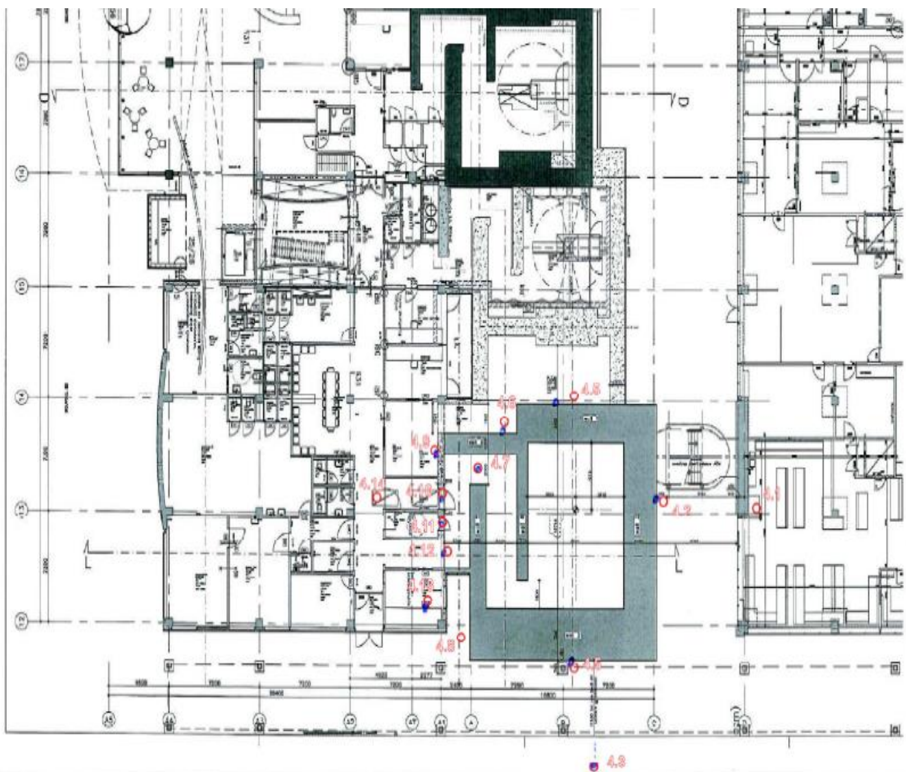
Figuur 1.4 Gedeelte van de plattegrond van de derde verdieping van MAASTRO Clinic/ ZON-PTC met aanduiding dosispunten. (technische tekening van Architecten aan de Maas)
