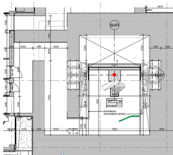
Figuur 2 Gedeelte van de plattegrond van het gelijkvloers van de bestralingsbunker ZON-PTC met aanduiding isocentrum en positie loodafscherming. (technische tekening van Architecten aan de Maas)
